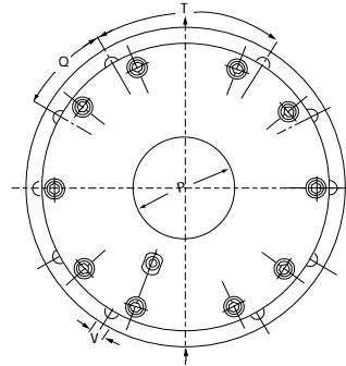
CSM Brake/Bremse
